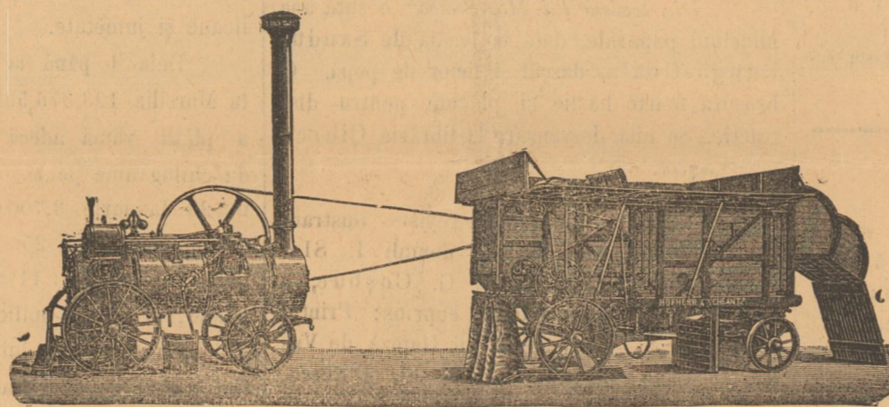
Garnitură de trier cu vapor.
