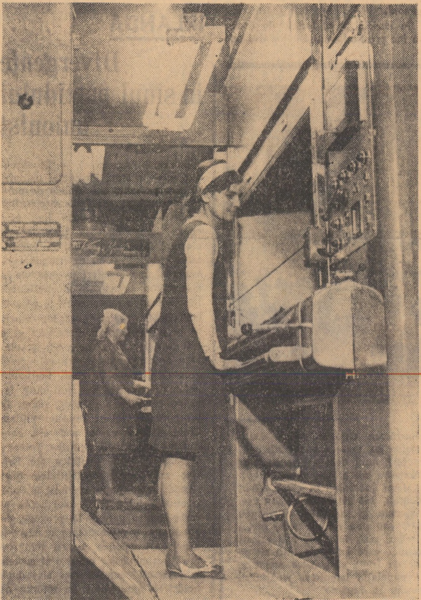
Cele două mașini de decatat din secția finisaj-apretură a fabricii „Libertatea” din Sibiu, care asigură o producție de bună calitate, realizează împreună apretarea a circa 6.000 metri stofă în 8 ore
