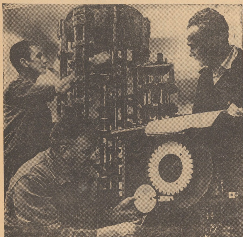
În atelierul aparatelor de comunicație al secției reparații mașini electrice de la I.R.E. Sibiu, o atenție deosebită se acordă recondiționării cutiilor de acționare a comutatoarelor pentru reglajul tensiunii la transformatori de mare putere
