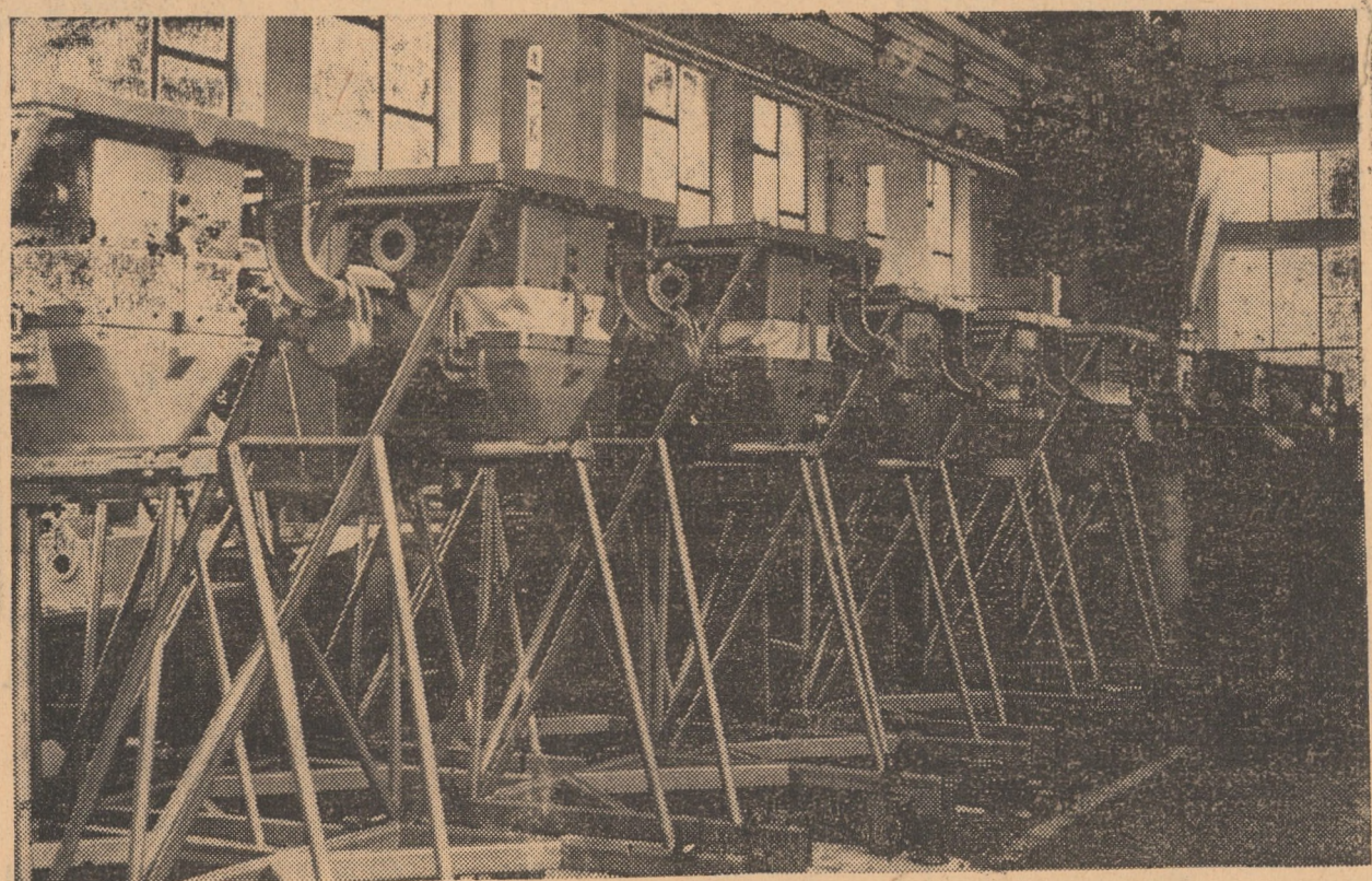
Înainte de-a fi expediat, o ultimă verificare a unui lot de balanțe de înscuit de 100 kg: produse destinate exportului, realizate de uzina „Balanța” din Sibiu.
