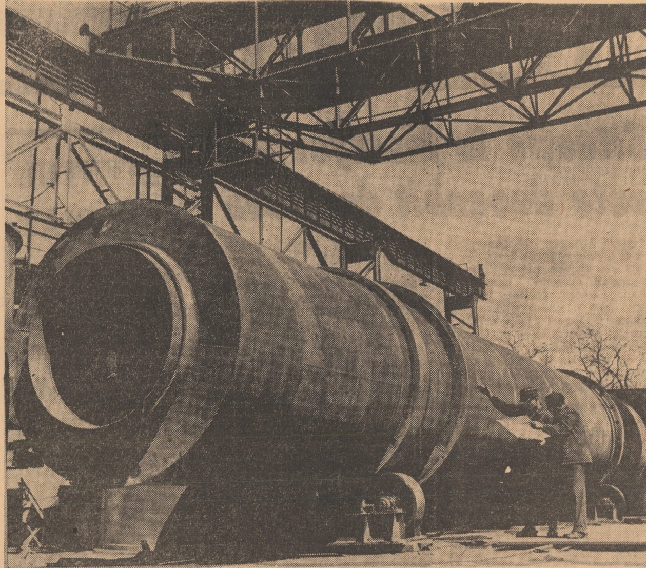
Granulator de mare tonaj pentru industria chimică, produs de uzina „Independența” Sibiu.
