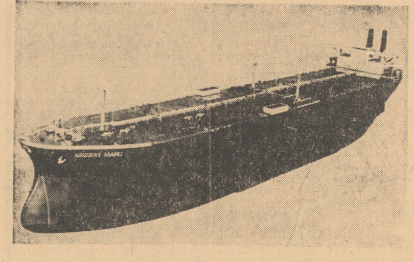
JAPONIA: Macheta celui mai mare petrolier din lume „Nisseki Maru” în construcție începînd din luna noiembrie la Șantierul naval din Kure. Petrolierul cu un deplasament de 372 400 tone, lung de 347 m, lat de 54,5 m, și adînc de 35 m poate dezvolta o viteză de 14,5 noduri, cu un motor de 40 000 de cai putere, va fi gata în noiembrie 1971. Capacitatea — 450 000 kilolitri la un transport.
