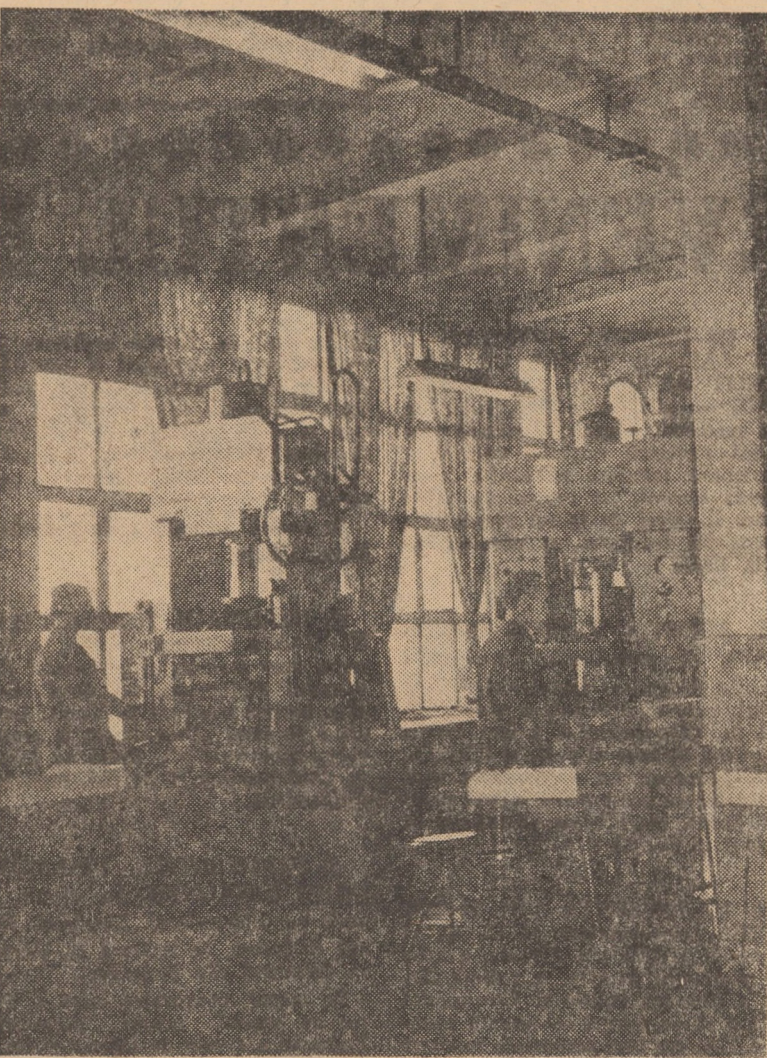
Secția termorigide în care se execută piese de schimb pentru industria ușoară: capace delco, minere geamantan, role pentru mașini de spălat rufe etc
