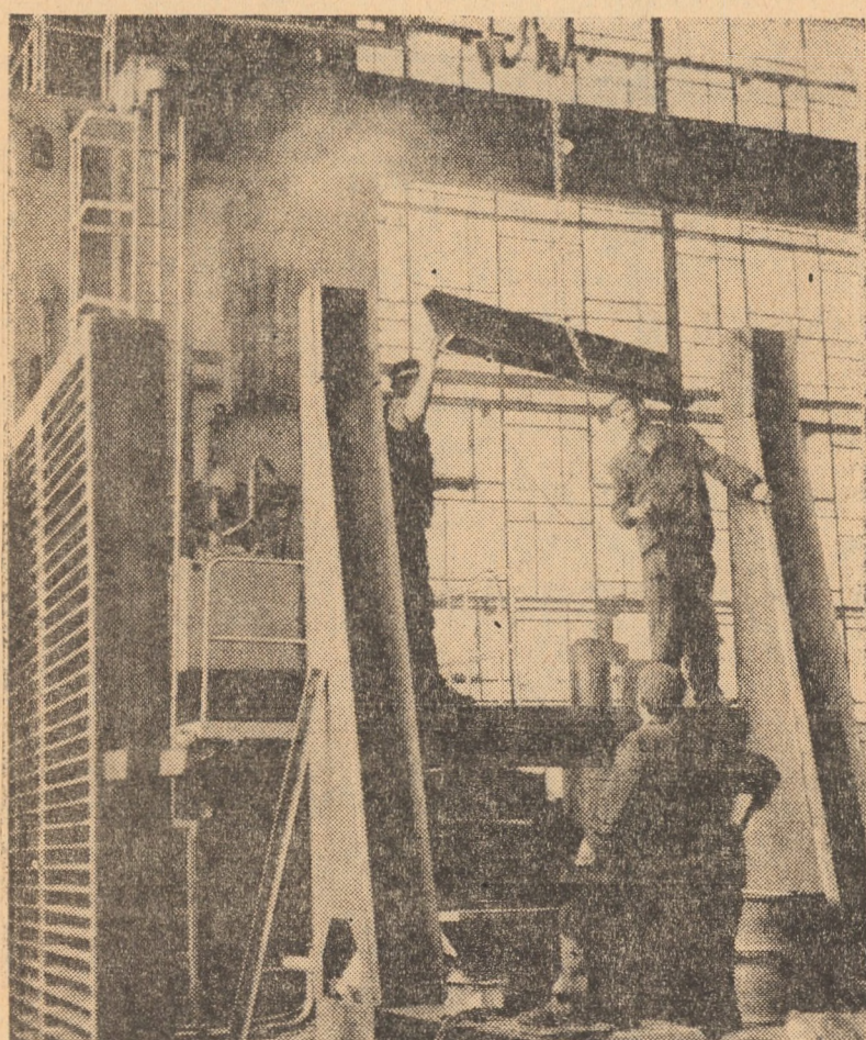
Lucrări de montaj la un cuptor cu inducție de 2,5 tone pentru turnătorii centrală din Cimpina, executat la uzina „Independența” din Sibiu
