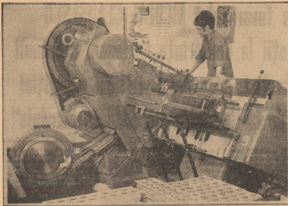
Unul din utilajele de mare productivitate din secția ambalaje metalice a F.P.C.C. „Salconserv” Medias; presa pentru ambutisat capace pentru cutiile de conserve deservită de tînrul comunist Ion Băcilă
