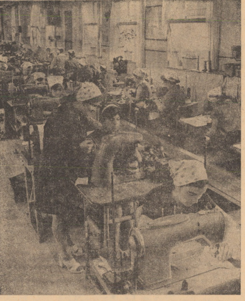
Unul dintre agregatele de confecționat încălțăminte cu deservire automată a locurilor de muncă de la I.P. Agnita
