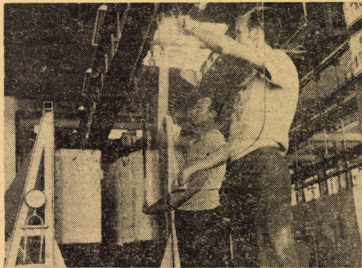
Întreprinderea de geamuri Mediaș: securizarea geamurilor curbate de parbriz pentru autocamionul ROMAN Diesel
