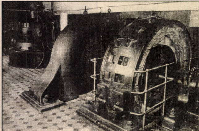
Producătorii de energie sibieni între astăzi și ieri: Hidrocentrala de la Gura Râului, încorporată în baraj și generatoarele de curent ale "bunicii" centralelor românești de la Uzina Sadu I
