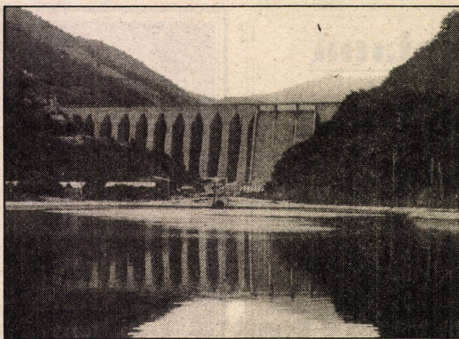
Producătorii de energie sibieni între astăzi și ieri: Hidrocentrala de la Gura Râului, încorporată în baraj și generatoarele de curent ale "bunicii" centralelor românești de la Uzina Sadu I
